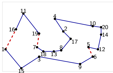
(a) ottimo locale: L = 319
