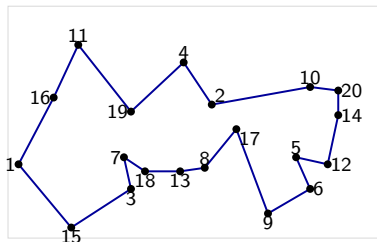
(c) dopo 2-opt: L = 303
