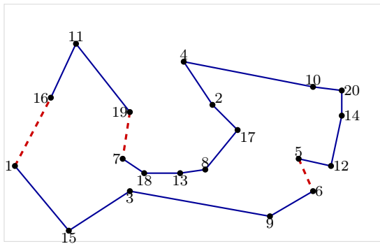
(a) ottimo locale: L = 319
