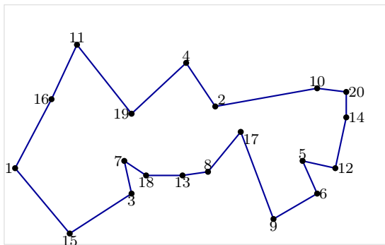
(c) dopo 2-opt: L = 303
