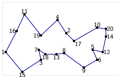
(d) after the second iteration: L = 291
